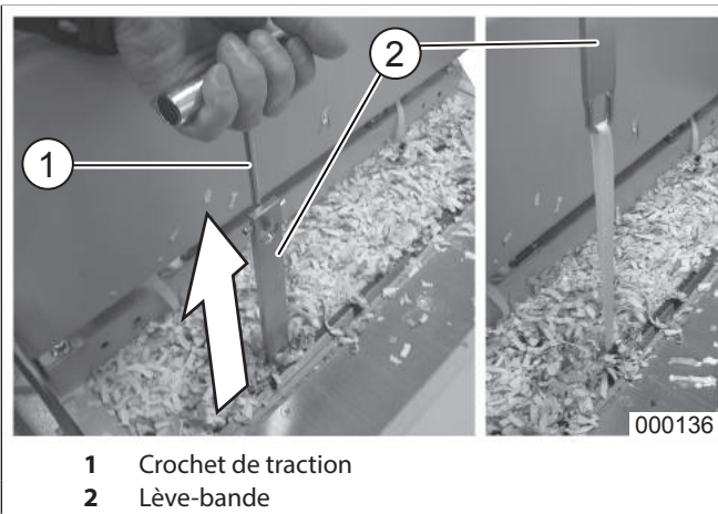
fig. 15 Lève-bande
