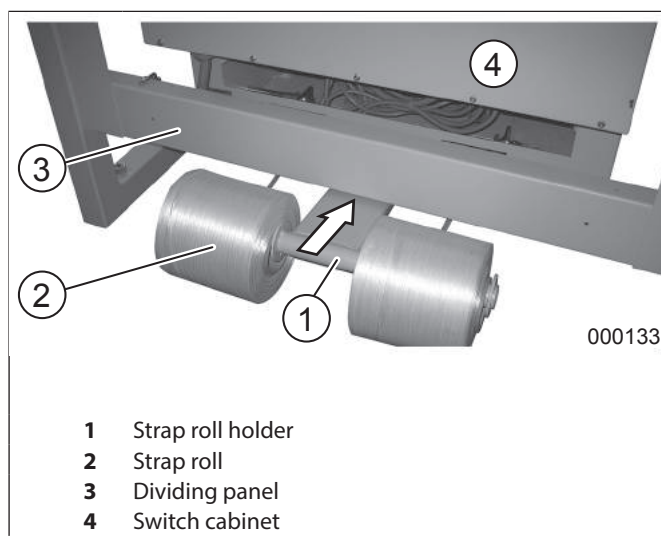
fig. 5 Strap rolls
