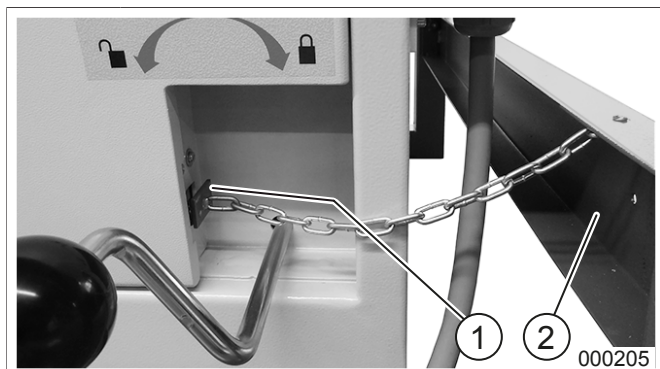
fig. 4 Verrouillage du fin de course
