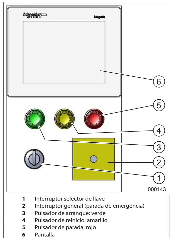
fig. 7 Elementos de manejo
