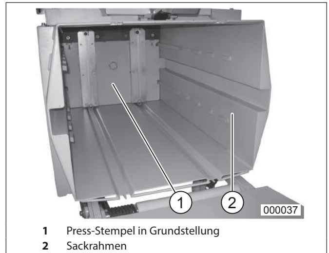
Abb. 13 Presse
