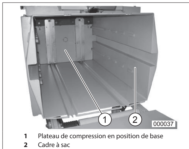
fig. 13 Presse
