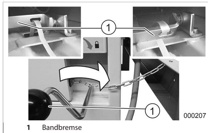
Abb. 14 Bandbremse
