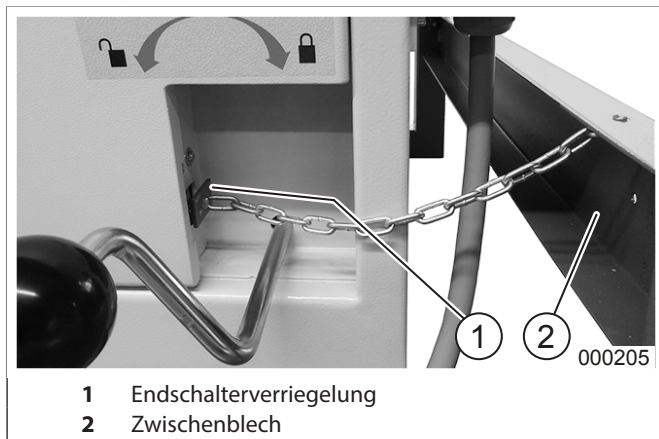
Abb. 4 Endschalterverriegelung
