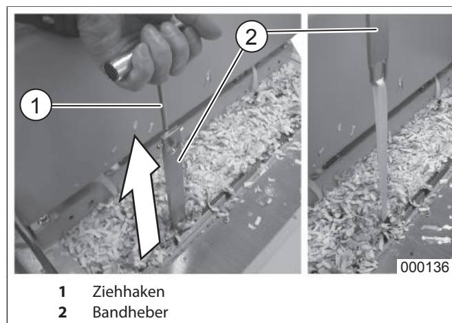
Abb. 15 Bandheber
