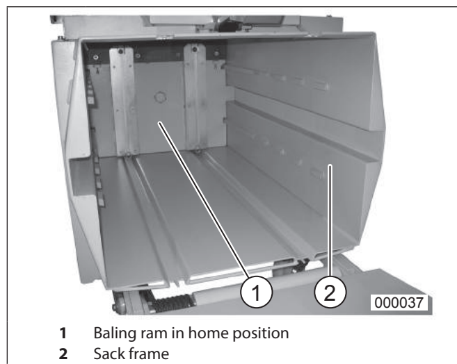
fig. 13 Baler
